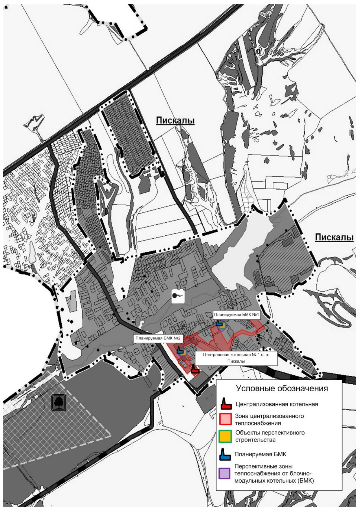
Рис. № 3 - Перспективные зоны теплоснабжения существующих систем теплоснабжения и источника тепловой энергии, планируемого к размещению на территории с. Пискалы
