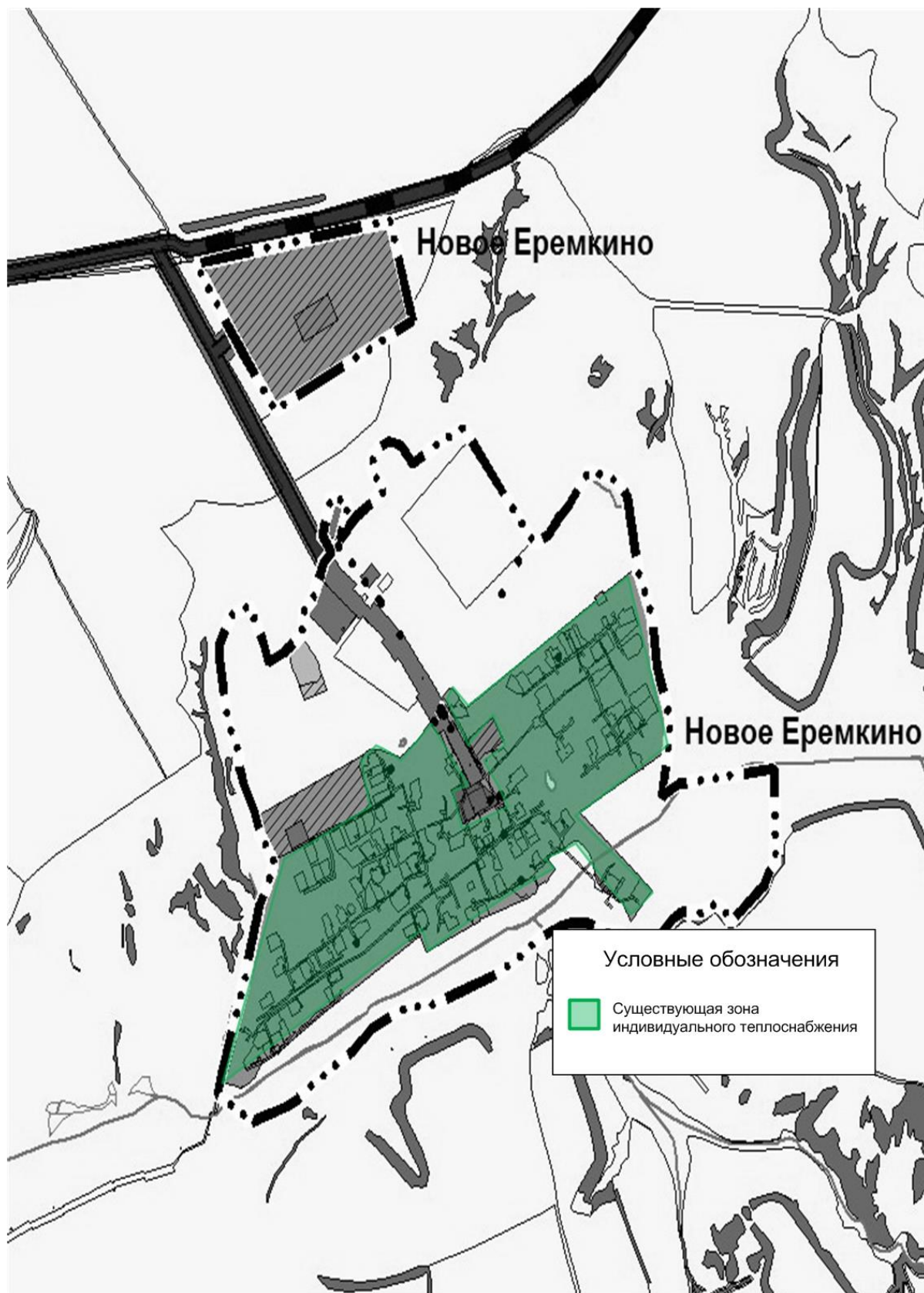
Рис. № 6 – Существующие и перспективные зоны действия индивидуальных источников тепловой энергии на территории поселка Новое Ерёмкино (развитие жилой зоны планируется в существующей застройке)
