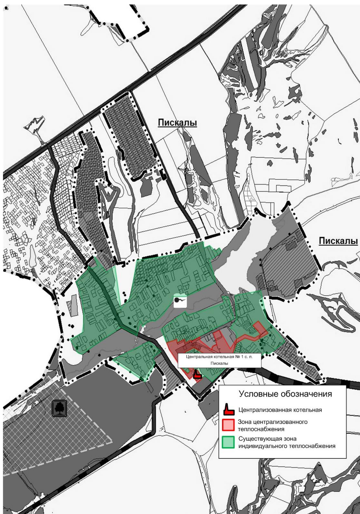
Рис. № 5 – Существующие и перспективные зоны действия индивидуальных источников тепловой энергии на территории поселка Пискалы (развитие жилой зоны планируется в существующей застройке)
