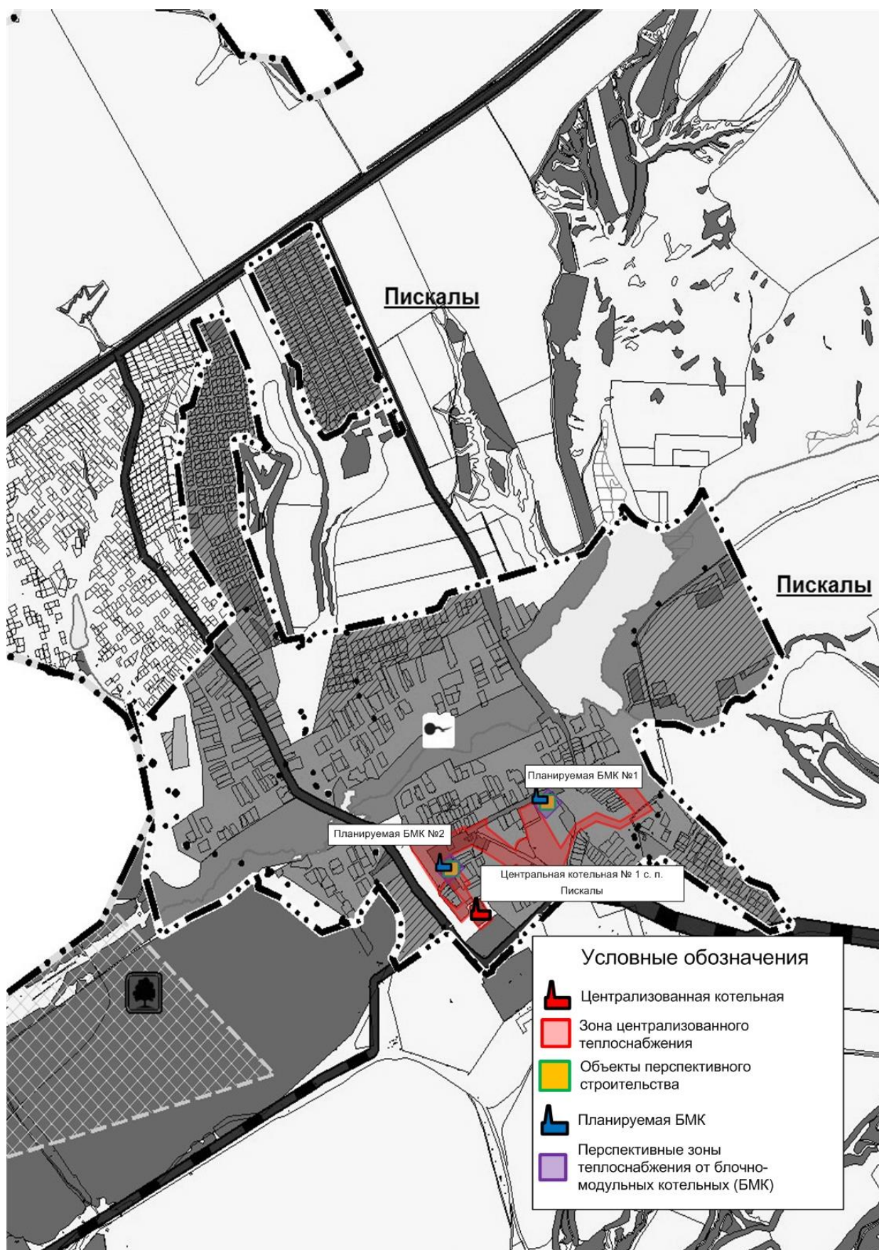
Рис. № 4 - Перспективные зоны теплоснабжения существующих систем теплоснабжения и источника тепловой энергии, планируемого к размещению на территории п. Пискалы
