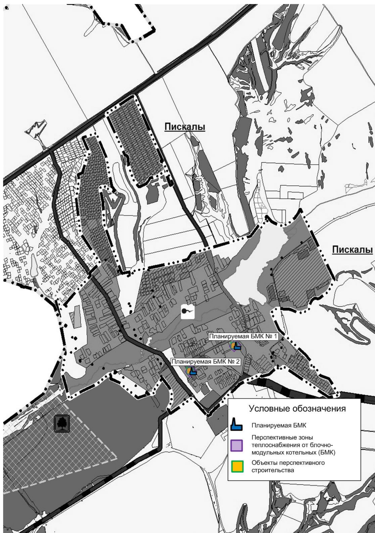
Рис. № 2.4 - Перспективные зоны теплоснабжения существующих систем теплоснабжения и источника тепловой энергии, планируемого к размещению на территории с. Пискалы
