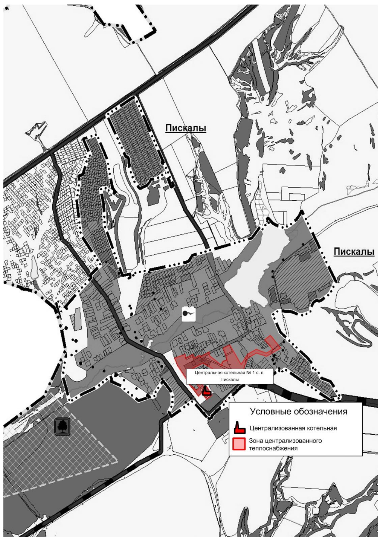
Рис. №1.4.1 - Зоны действия независимых систем теплоснабжения на базе локальных котельной на территории села Пискалы
